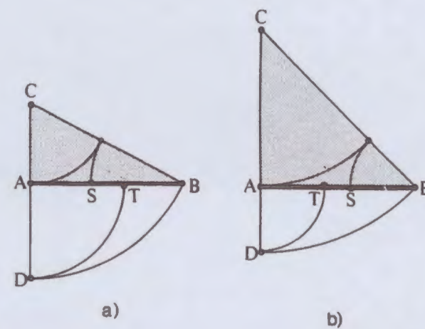
Figur 183. a) Teilung im Modulus \phi und b) im Modulus \sigma .
