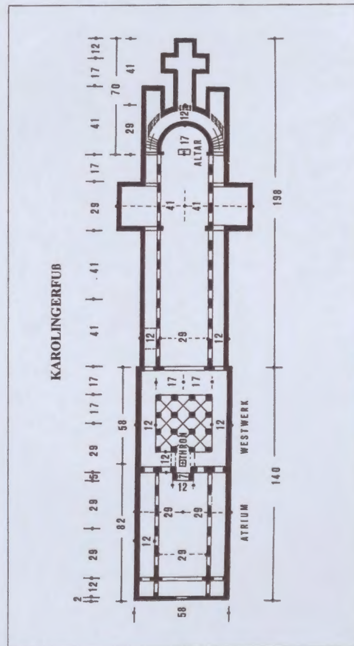
Figur 59: Der Tempel von Corvey besteht aus einem Atrium, einem »Westwerk«, der dreischiffigen Basilika und einer Umgangs-krypta. Mit Hilfe der Idealzahlen und mit dem »Karolingerfuß« als neuer Maßeinheit konnten die Vorgaben der biblischen Prophe-zeiungen realisiert werden.
