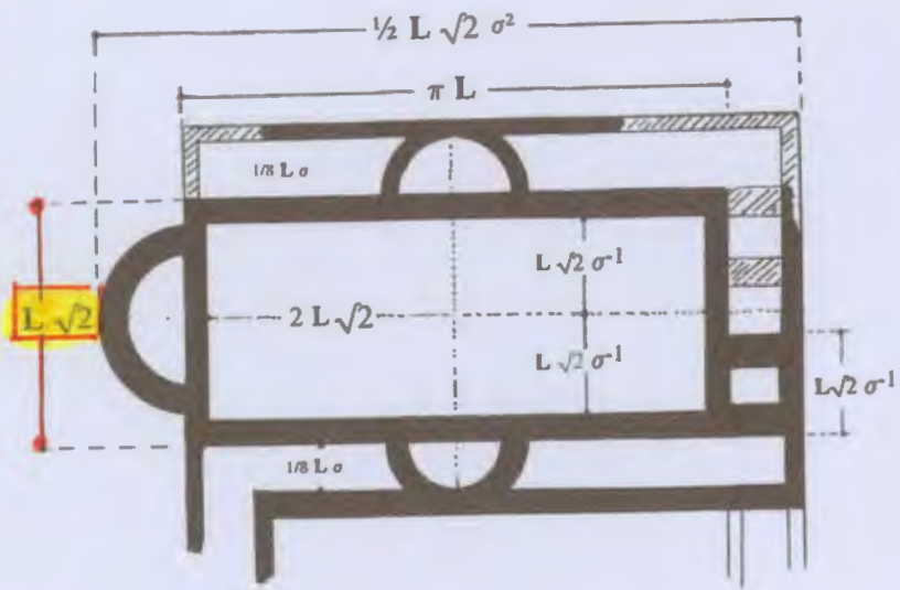
Figur 16. Idealgrundriss der Königshalle am Ort des heutigen Rathauses mit drei Apsiden. Im Osten stand der Granus-Turm als Treppenhaus zum Obergeschoss der Königshalle. S. 67
