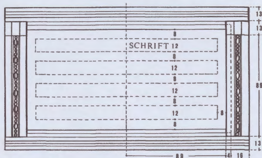
Figur 63: Eine genauere Analyse der Maße enthüllt die Verwendung der Maßeinheit » 1/2 Fingerbreite« und der Heiligen Zahlen . Der Grund dafür ist die Verwendung der römischen CAPITALIS QUADRATA als Schrift.
