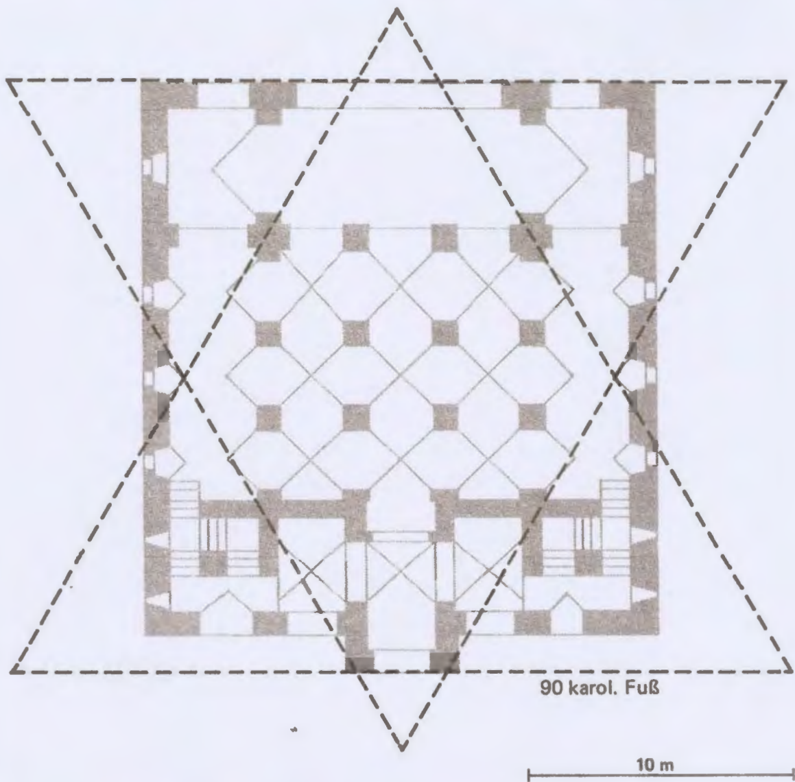
Zeichn. 6: Grundriß des Corveyer Westwerks. Das eingezeichnete Dreieck von 90 karol. Fuß Seitenlänge ist das Ausgangsdreieck der in Zeichnung 5 abgebildeten Dreieckskette.
