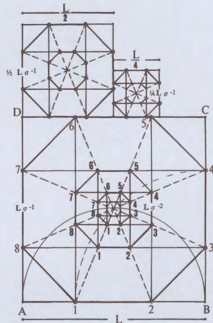
Figur 164. Die in Aachen verwendeten Maßlängen erhält man am einfachsten aus selbstähnlichen Achtecken, die mit dem Idealschnitt in Quadraten mit Seitenlängen von L ; L/2 ; L/4 ; L/8 ; L/16 \dots konstruiert wurden.
