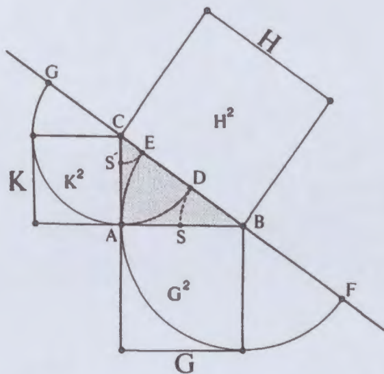
Figur 181. Allgemeiner Schnitt am rechtwinkligen Dreieck.
