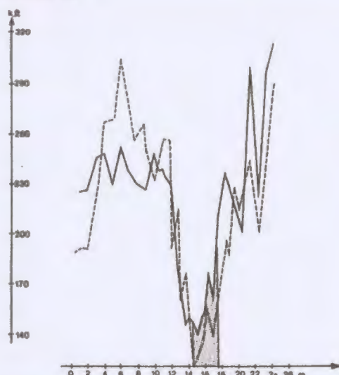
Verlauf des Bodenwiderstandes über einem Reizstreifen
