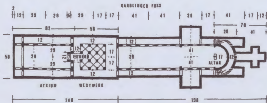
Figur 169. Die Kirche von Corvey bestand aus Atrium, Kaiserhalle (Westwerk), Längs- und Querschiff, Allerheiligstem mit Umgangschor und einer kreuzförmigen Apsis.
