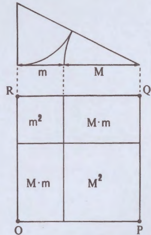
Figur 189. Unsymmetrische Flächenteilung eines Quadrates durch den Goldenen Schnitt.
