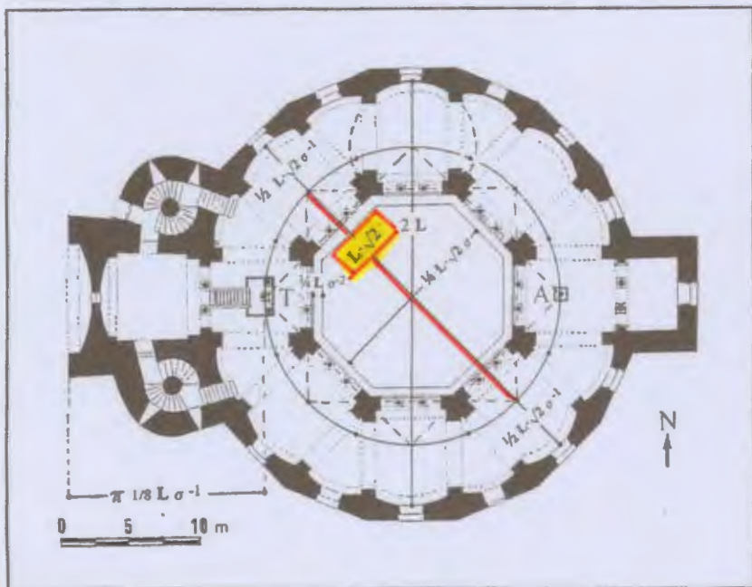
Figur 16. Idealgrundriss der Königshalle am Ort des heutigen Rathauses mit drei Apsiden. Im Osten stand der Granus-Turm als Treppenhaus zum Obergeschoss der Königshalle. S. 67
