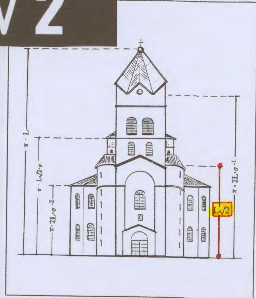
Figur 29. Rekonstruktionsvorschlag für den Turm im Westen des Zentralbaus. Das gefaltete Zeltdach berücksichtigt die Darstellung auf dem staufischen Karlsschrein. Seite 89
