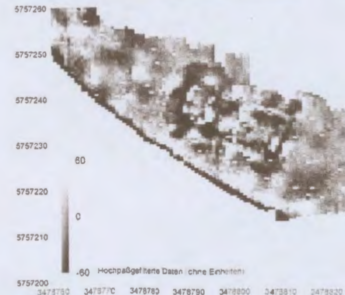
Abb. 13 b: Fundamente eines sächsischen Vorläuferbaus
