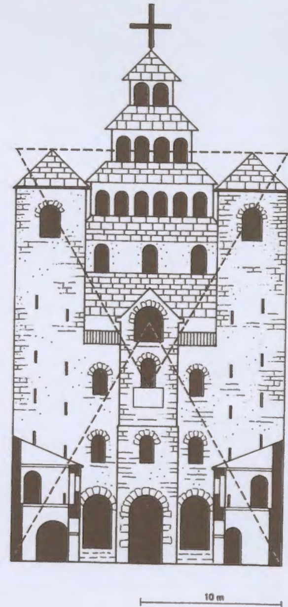
Zeichn. 8: Das vierte Dreieck der Dreieckskette (Zeichn. 5) in die rekonstruierte Westwerkfassade doppelt eingezeichnet. Bemerkenswert ist, daß durch die Überlagerung der beiden Dreiecke gerade dort eine Raute (vgl. Abb. 8) entsteht, wo auch schon die Dreieckspitzen allein eine Beziehung zum Kaiser erkennen lassen.
