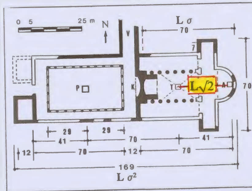
Figur 10. Grundriss der Pippin-Basilika mit den schwarz gezeichneten Fundamentresten, die sich von ihr erhalten haben. Die Kirche hatte die Gestalt eines ägyptischen Kreuzes mit vorgelagertem Atrium. In der Mitte der Anlage mündete von Norden her der Verbindungsgang in eine Vorhalle. Die Gesamtlänge der Kirchenanlage in Ost-Westrichtung betrug 150 Fuß. S. 39
