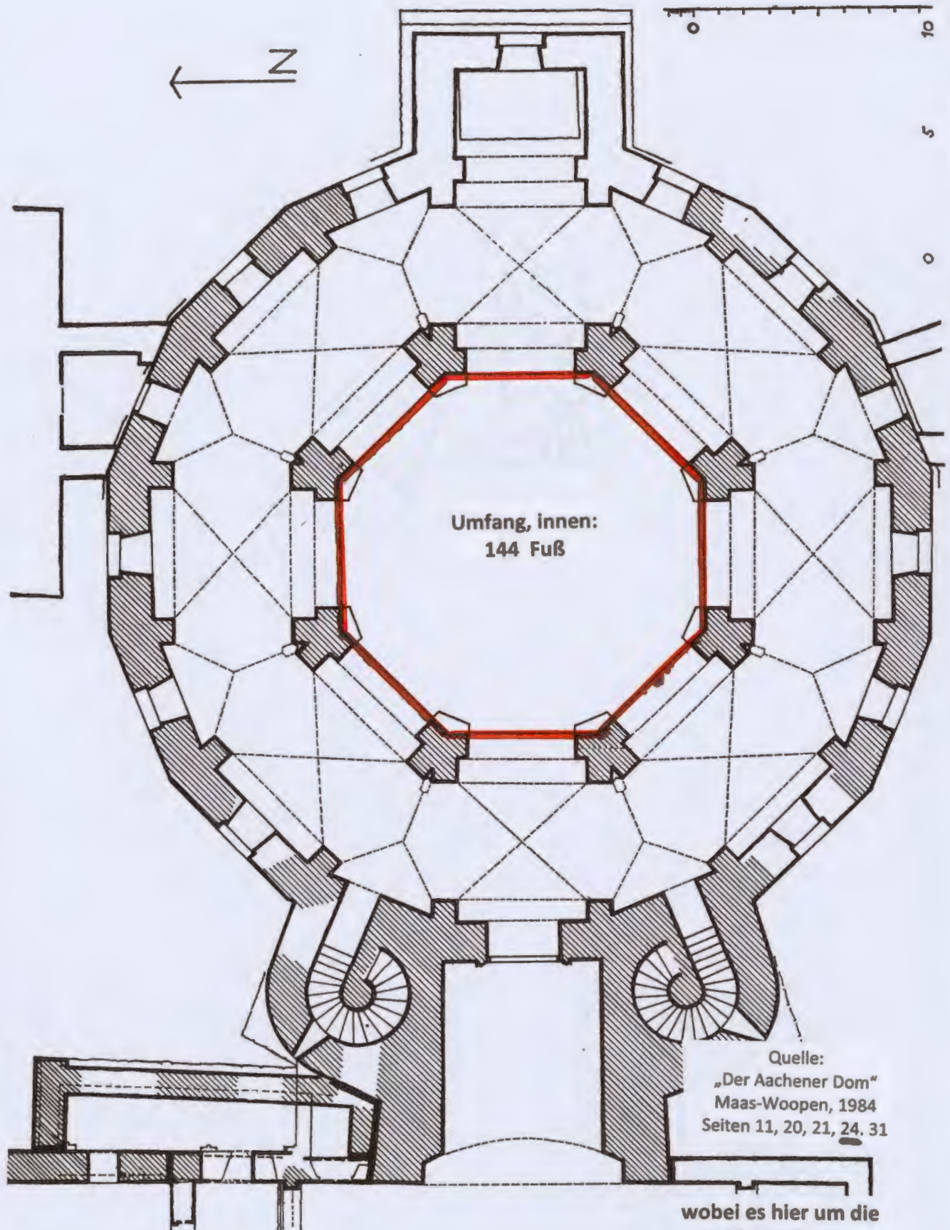
Pfalzkapelle, Grundriß des Erdgeschosses; im Osten Rekonstruktion des karolingischen Chores (Kreusch 1965, geringfügig verändert)
