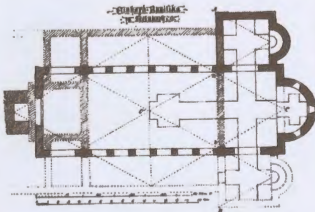
Die Triangulation nach C. Alhard von Drach (1897) mit gleichseitigen Dreiecken
