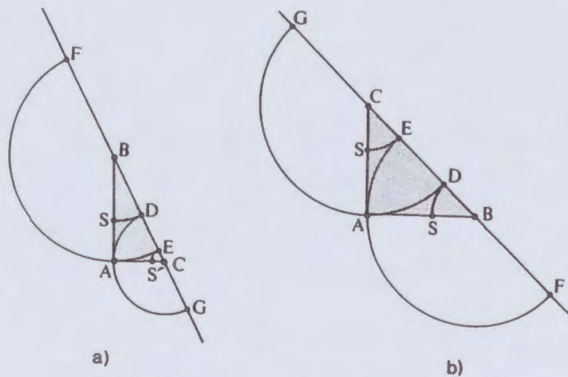
Figur 182. Goldener Schnitt a) und Idealschnitt b) am rechtwinkligen Dreieck.
