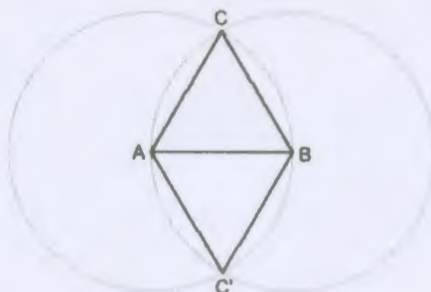
Gleichseitiges Dreieck, Seitenlänge vorgegeben
