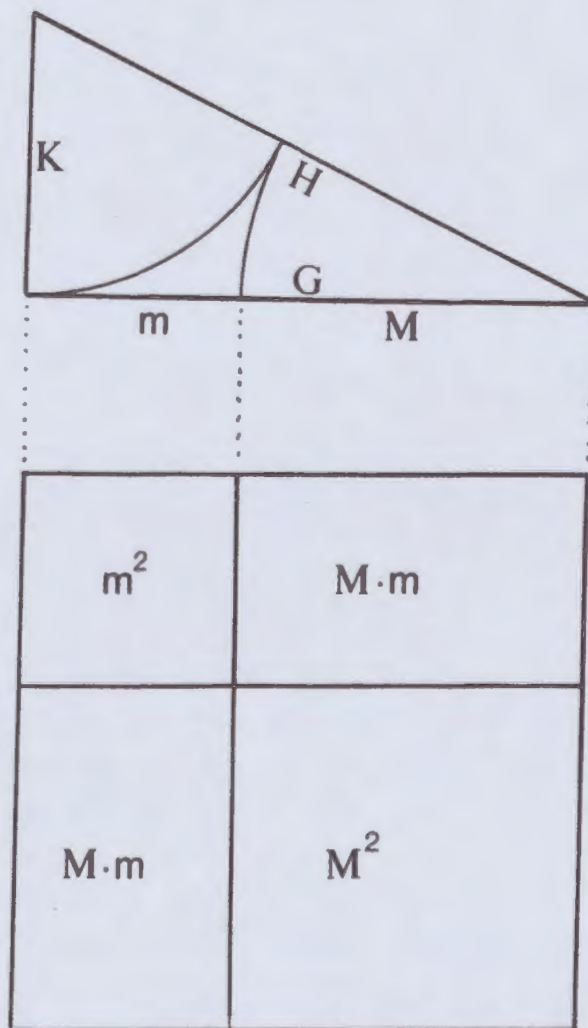
Figur II Der »Goldene Schnitt« unterteilt die große Kathete G in Major ( M ) und Minor ( m ). Es verhalten sich (M + m) : M wie M : m . Das irrationale Verhältnis hat den Wert \Phi . Die Seitenteilung eines Quadrates führt auch zur Flächenteilung im Verhältnis \Phi . Die Flächendifferenz M^2 - m^2 hat denselben Wert wie die Fläche eines »Goldenen Rechtecks« M \cdot m .
