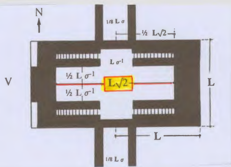
Figur 17. Die Fundamente des Torbauwerks wurden mit der Breite L und der Länge 2L geplant. In den Obergeschossen, zu denen mehrere Treppenhäuser hinaufführten, waren die kaiserlichen Gemächer untergebracht. S. 68
