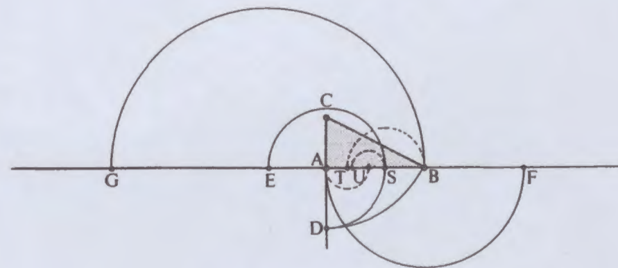
Figur 184. Vergrößerung einer beliebigen Strecke AB mit dem Modulus \phi .
